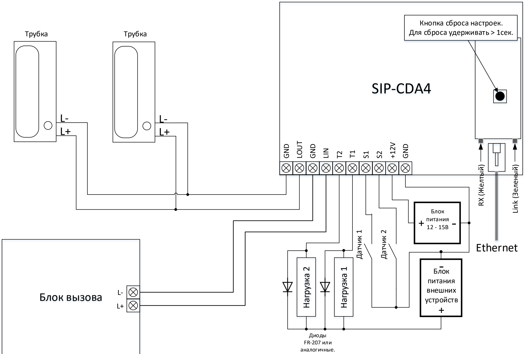
Схема подключения SIP-CDA4.
